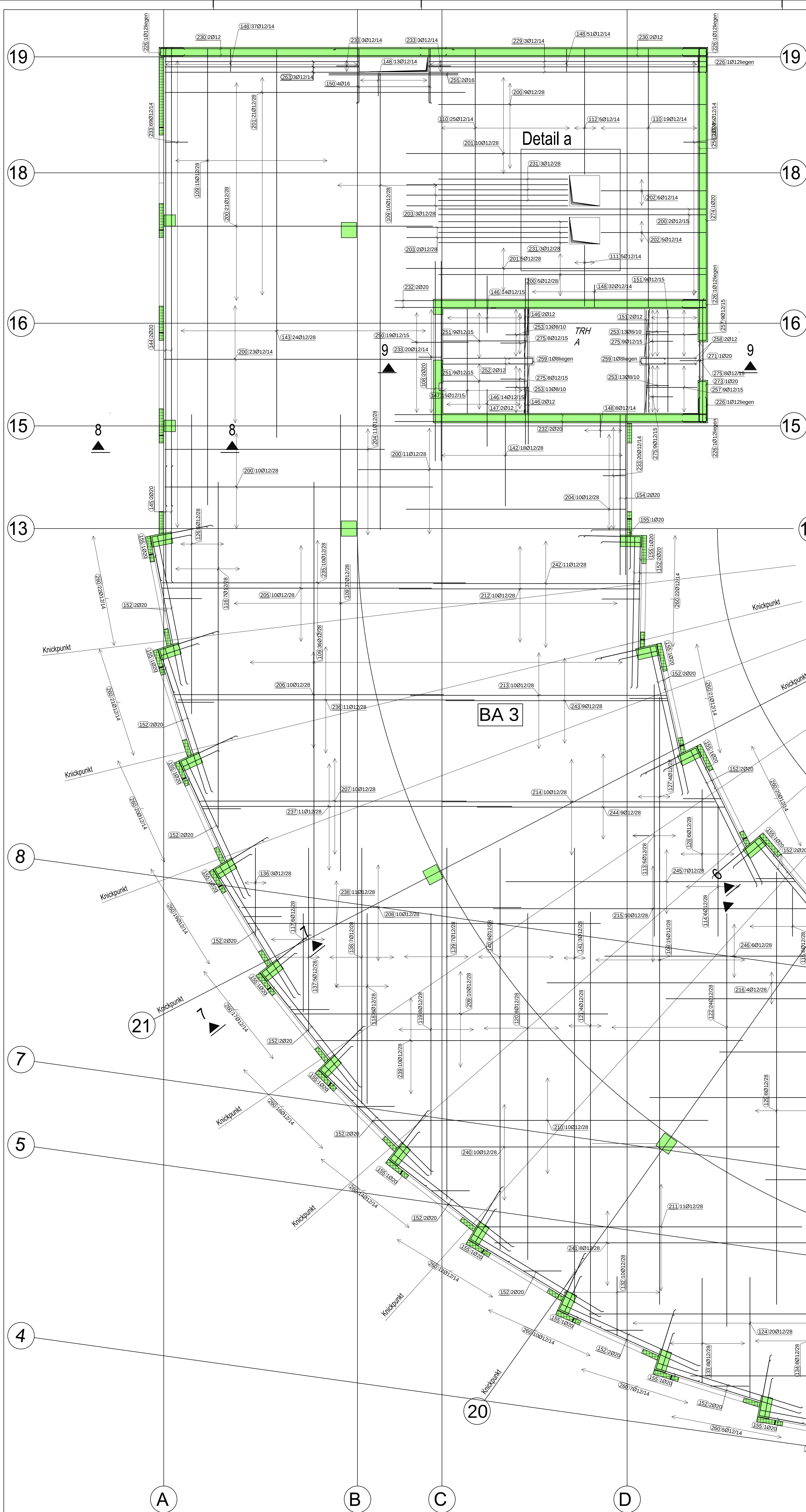
Grundriss 1.Obergeschoss BA 3 - untere Lage und Schnitte M 1:50
